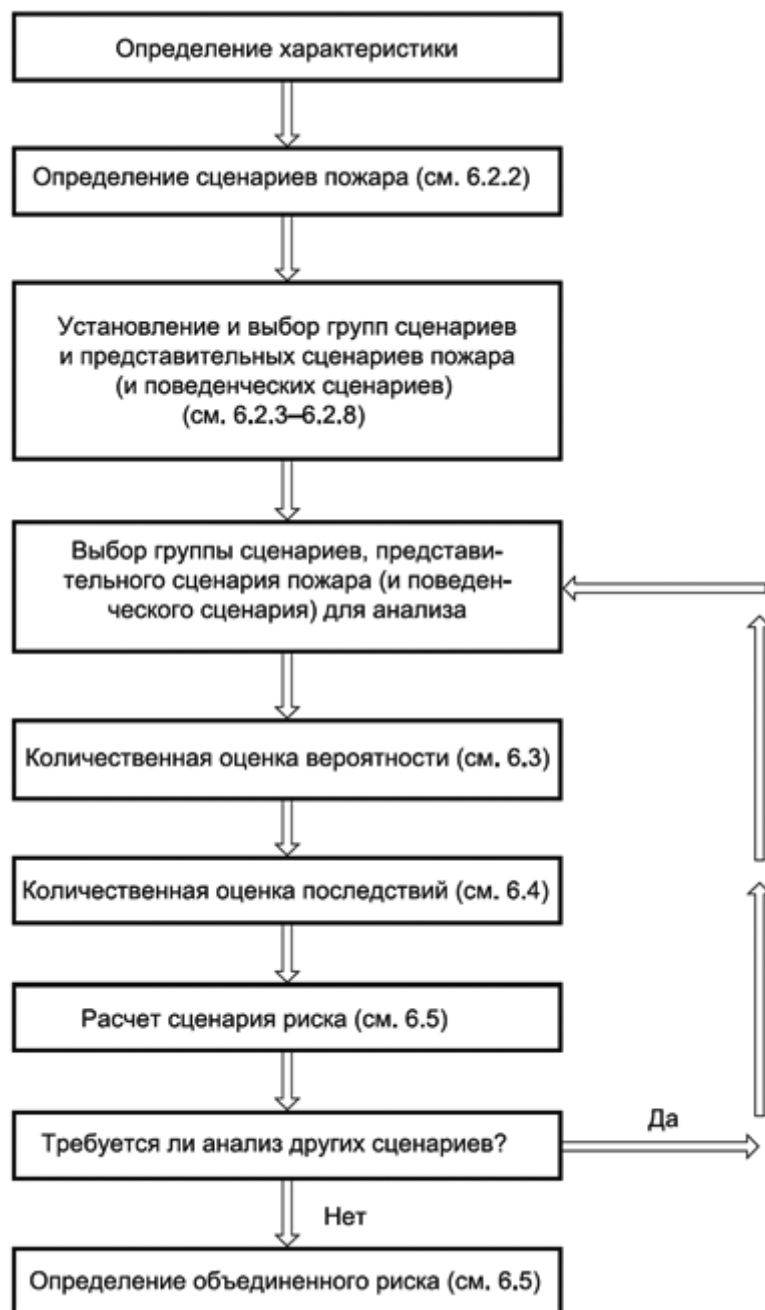
Рисунок 2 - Схема оценки пожарного риска
